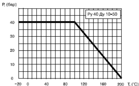
Зависимость «Температура-Давление»
