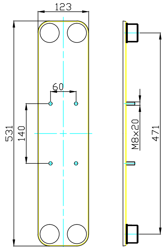
NB-533 Optional stud bolt placement 60x291mm
